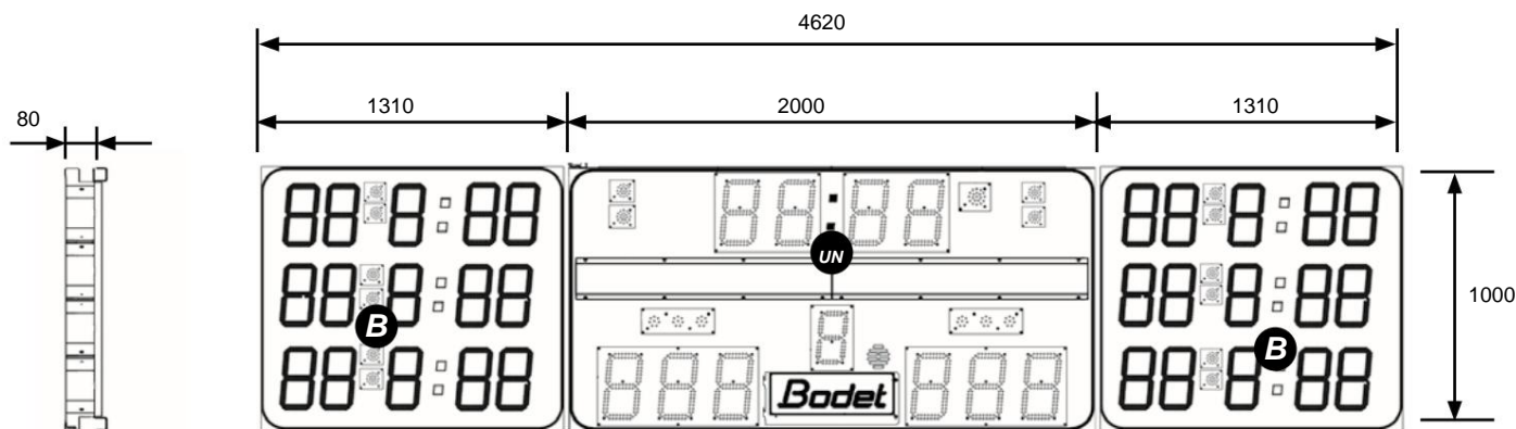
Vista laterale
