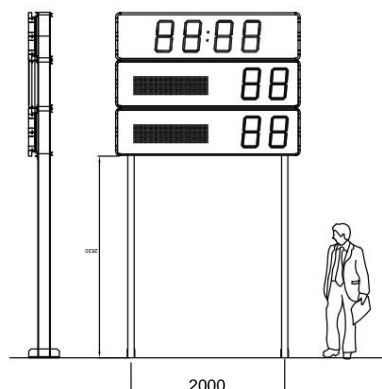
Supporto BT2045 Alfa
