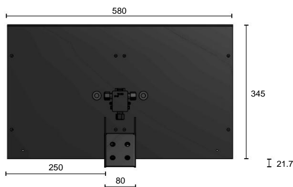
Pannello solare vista dal basso:
