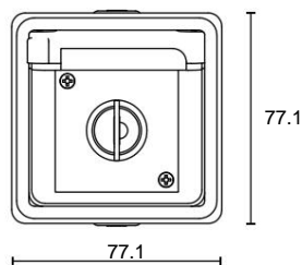
Interruttore a chiave vista frontale:
