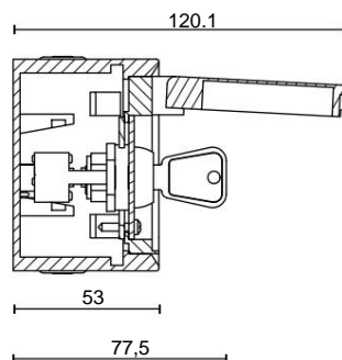
Vista laterale dell'interruttore a chiave:
