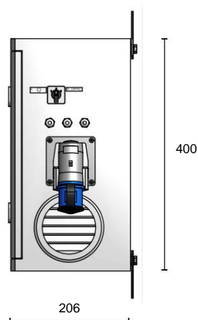
Vista laterale armadio:
